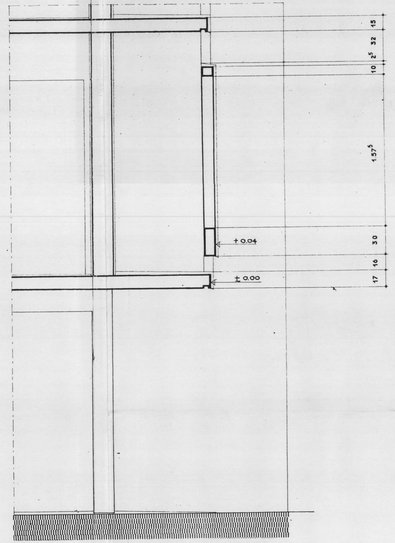
COUPE SUR LOGGIA EN PIGNON OUEST DU BATIMENT A
